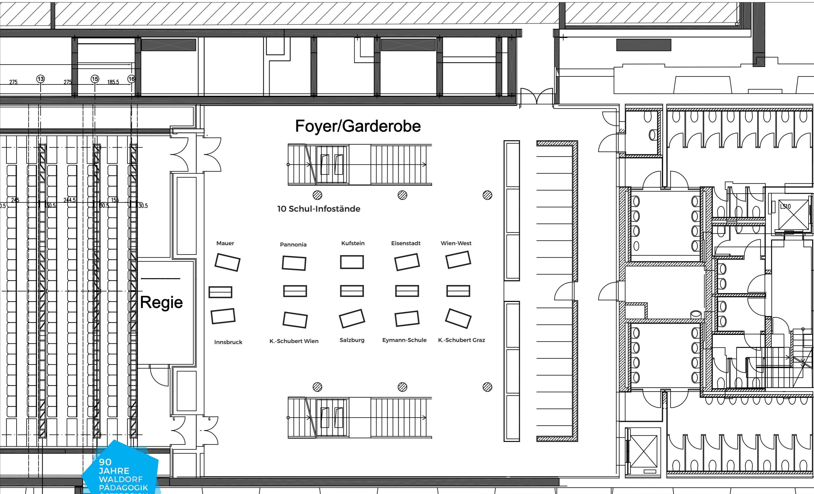
90 JAHRE WALDORFPÄDAGOGIK MQ, HALLE G und Vorhalle/Foyer, GRUNDRISS M 1:100
